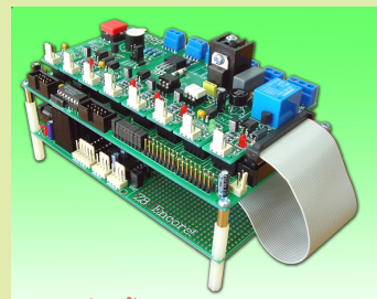
รูปการต่อใช้งาน ET-BUS I/O และชุด I/O MODULE เข้ากับบอร์ดคอนโทรลต่างๆ ของ อีทีที โดยต่อผ่านทาง PORT 34 PIN ET I/O BUS, 10 PIN ET BUS หรือ 10 PIN I 2 C BUS
