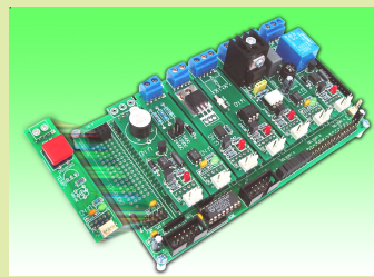
รูปการต่อใช้งาน ET-BUS I/O กับชุด I/O MODULE สามารถต่อขยาย I/O MODULE ได้ 8 ช่อง INPUT/OUTPUT
