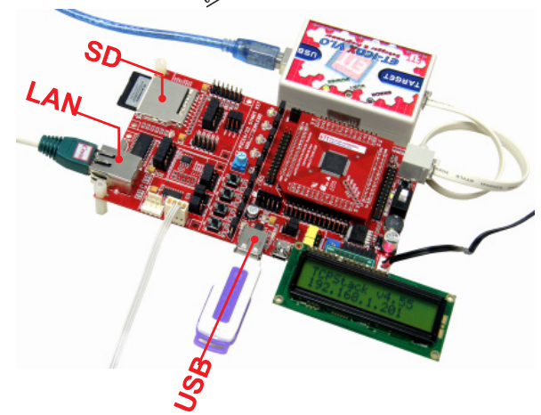
การต่อ ETT-PLUG IN MODULE MICROCHIPS เข้ากับบอร์ด ET-PIC16/32 START KIT
